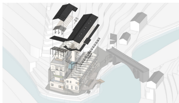
图12. 小桥流水人家轴侧示意图（来源：九七华夏KAI建筑工作室）
