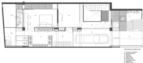
图9. KHouse平面图（来源：KC Design Studio）
